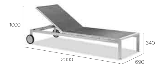
Lounge _ 647251 Shown at: P 265
