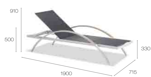
Lounge _ 653051 Shown at: P 263
