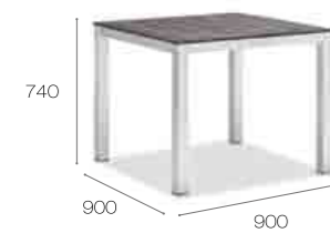
Square Dining Table_ 807771 Shown at: P 292
