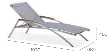
Lounge _ 811751 Shown at: P 222
