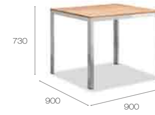
Square Dining Table _ 800171 Shown at: P 211
